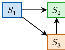
Condensation (DAG)
