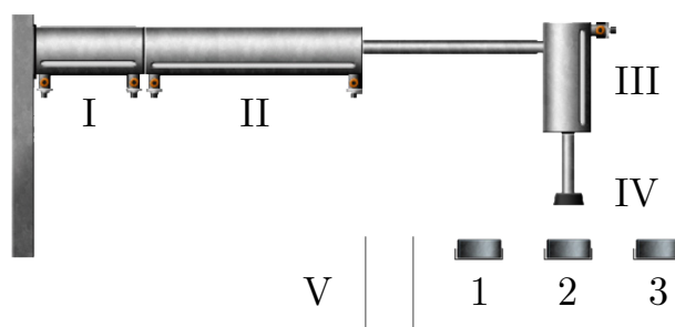
Рисунок 8 — Pick-and-Place манипулятор
